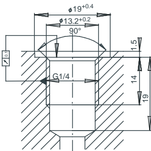
G 1/4 DIN 3852-E
