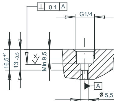
G 1/4
