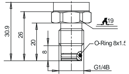
G 1/4 B
