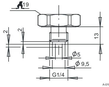
G 1/4 B EN 837
