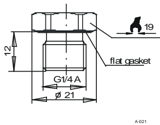
G 1/4 A DIN 3852 -E
