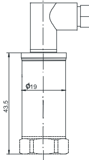
plug DIN 43650 C
